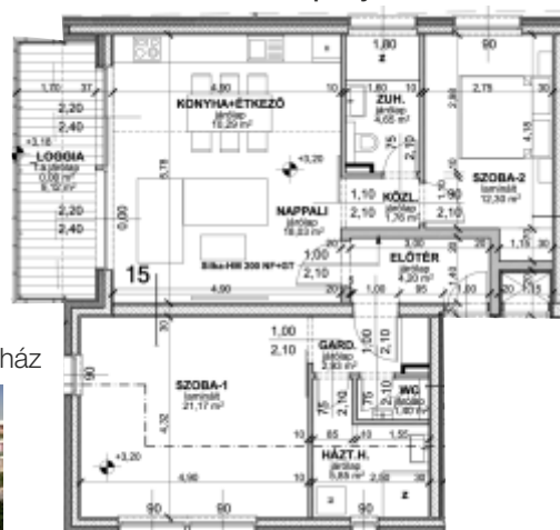
Műszaki alaprajz
